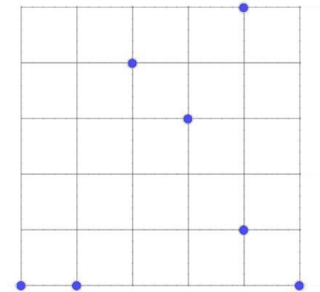
TRIANGOLO RETTANGOLO
