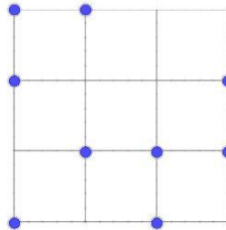
RETTANGOLO
