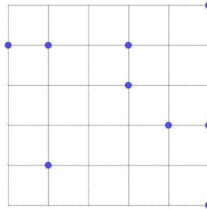
PARALLELOGRAMMA
